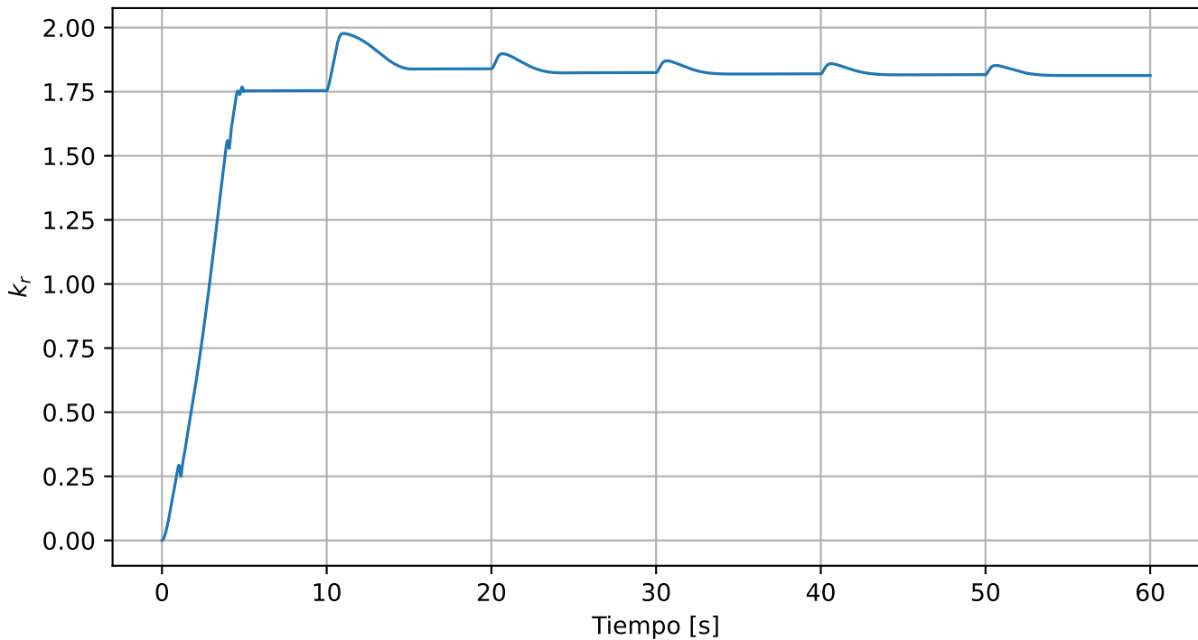
Evolución de k_r - tren de pulsos
